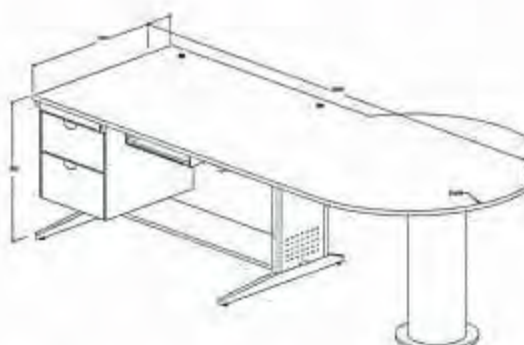
CP-2280/LP/POUT 體積 Size(mm):W2200*D800*H760
