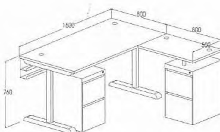
TL-1680/RSD 體積 Size: W1600*D800*H760mm TL-1880/RSD 體積 Size: W1800*D800*H760mm
