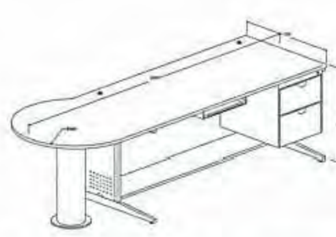
CP-2270/RP/POUT 體積 Size(mm):W2200*D700*H760
