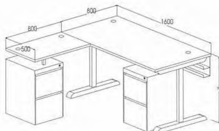
TL-1680/LSD 體積 Size: W1600*D800*H760mm TL-1880/LSD 體積 Size: W1800*D800*H760mm
