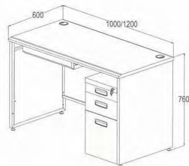
CW118-1060/RP 體積 Size: W1000*D600*H760mm CW118-1260/RP 體積 Size: W1200*D600*H760mm
