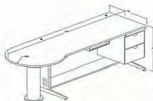
CP-2270/RP/PIN 體積 Size(mm):W2200*D700*H760
