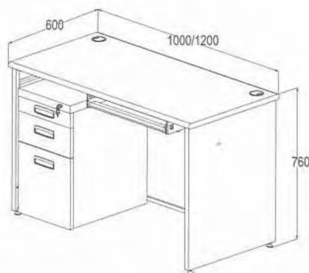
CW118-1060/LP 體積 Size: W1000*D600*H760mm CW118-1260/LP 體積 Size: W1200*D600*H760mm
