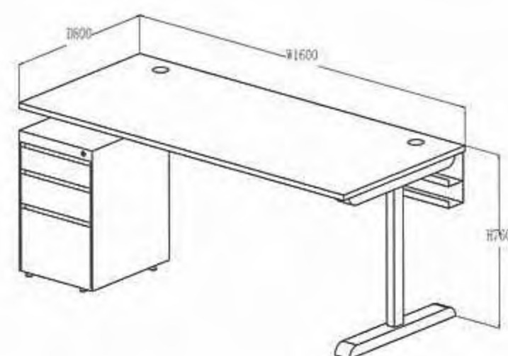
TL-1260 體積 Size: W1200*D600*H760mm TL-1470 體積 Size: W1400*D700*H760mm TL-1570 體積 Size: W1500*D700*H760mm
